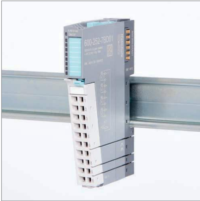
AI 4 x U, \pm 10 V, 0–10 V, 1–5 V, Iso., 16 Bit
